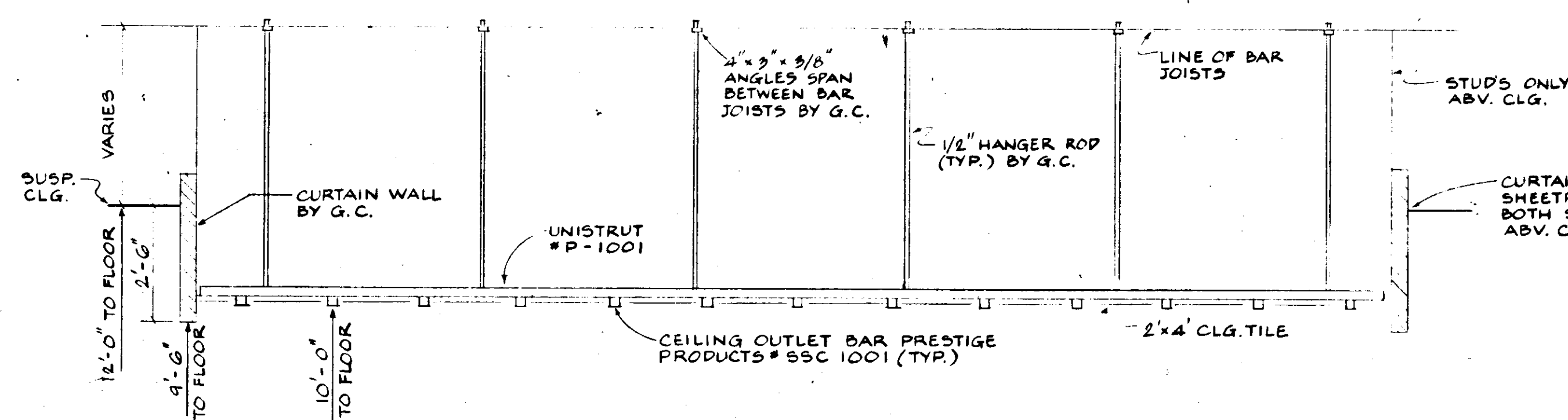
SECTION A-A' SCALE: 3/8" = 1'-0"
