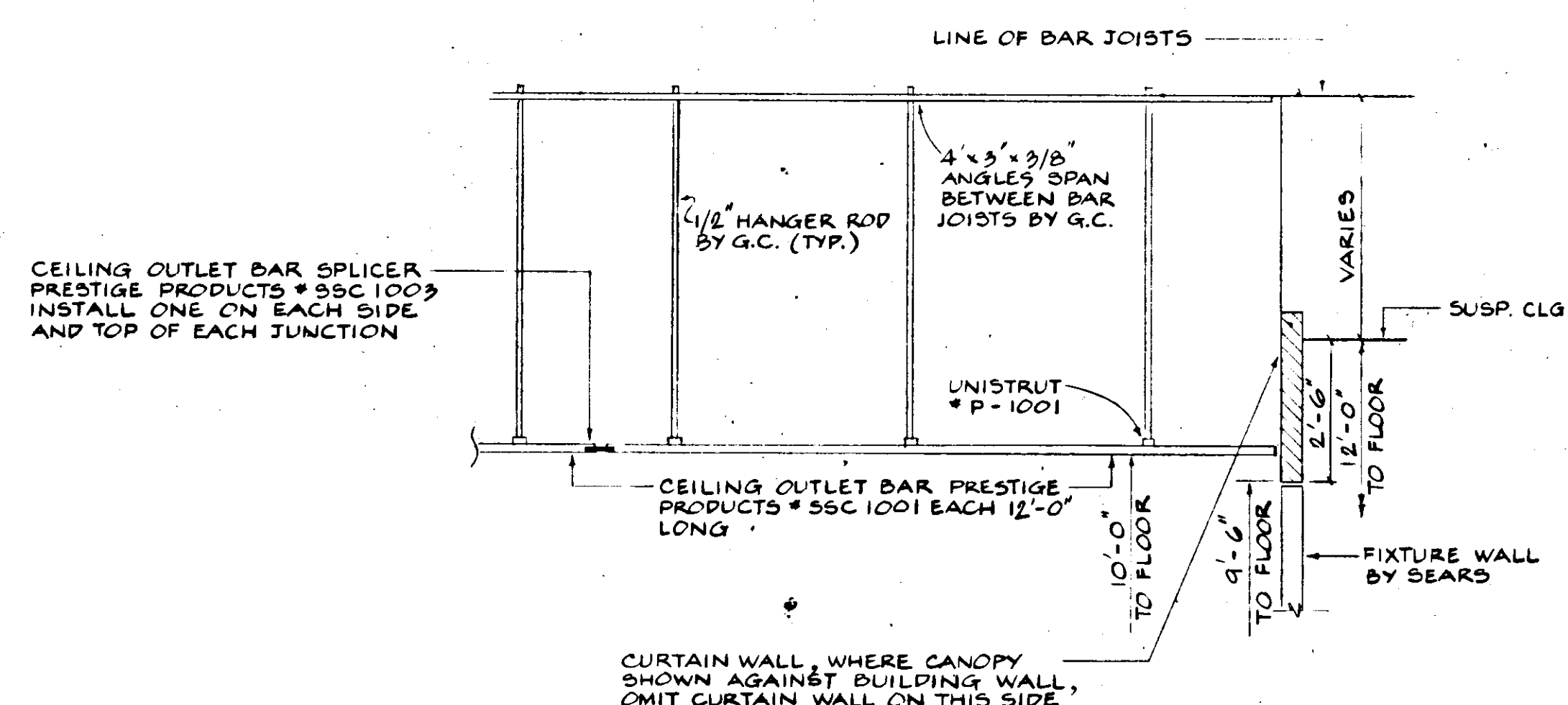
SECTION B-B' SCALE: 3/8" = 1'-0"
