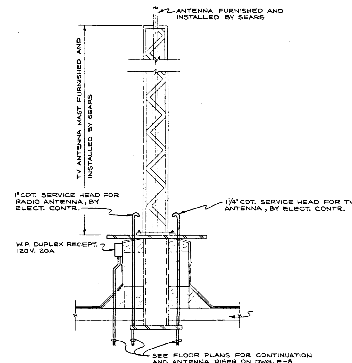
RADIO & T.V. ANTENNA POLE
