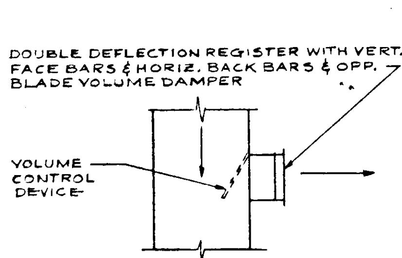
TYP. SIDE OUTLET SUPPLY DET. NO SCALE
