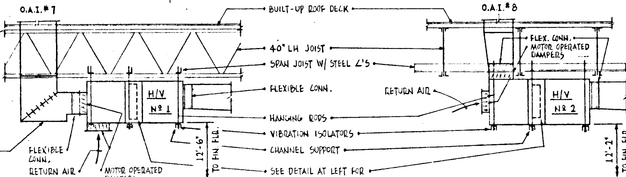
SECTION A-3 SCALE: 1/4" = 1'-0"
