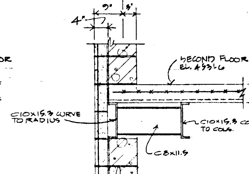
SECTION 5 SCALE: 1/2" = 1'-0"
