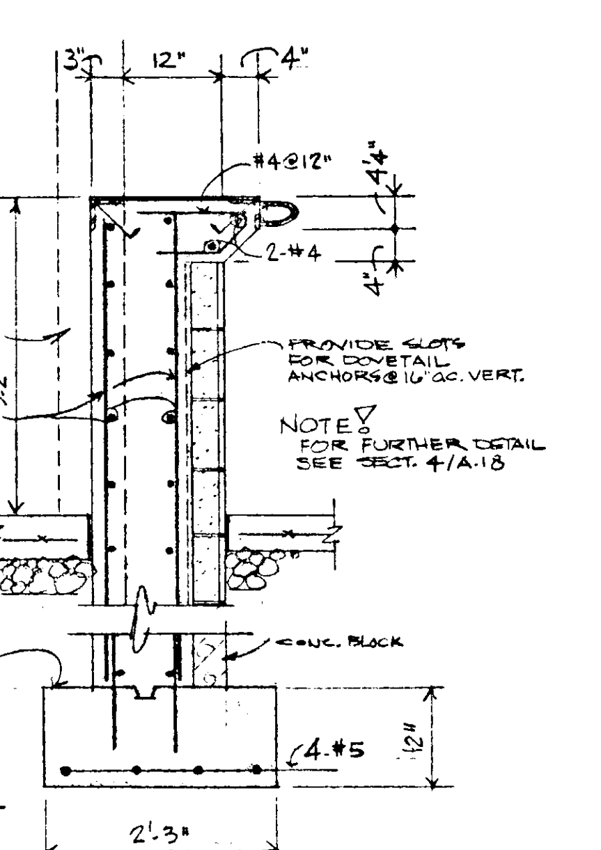
SECTION 14 SCALE: 1/2" = 1'-0"
