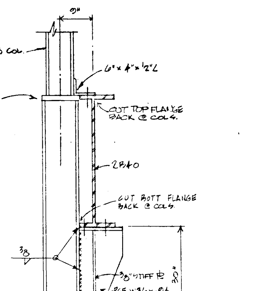
SECTION 6 SCALE: 1/2" = 1'-0"
