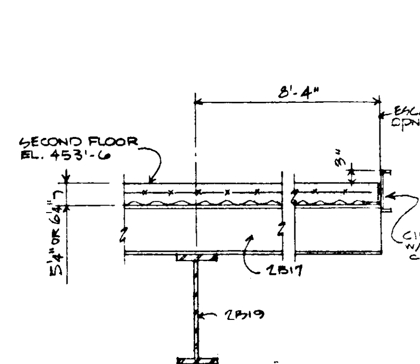
SECTION 1 SCALE: 1/2" = 1'-0"
