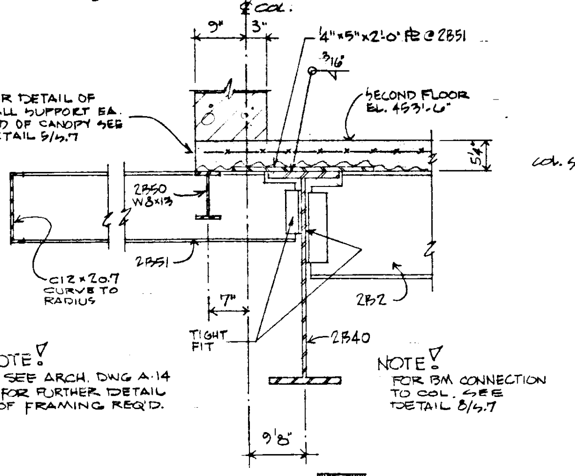
SECTION 4 SCALE: 1/2" = 1'-0"
